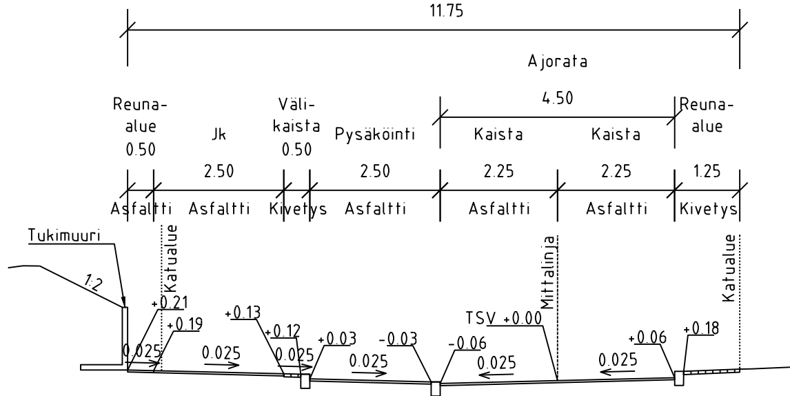
TYYPPIPOIKKILEIKKAUS B-B 1:100
