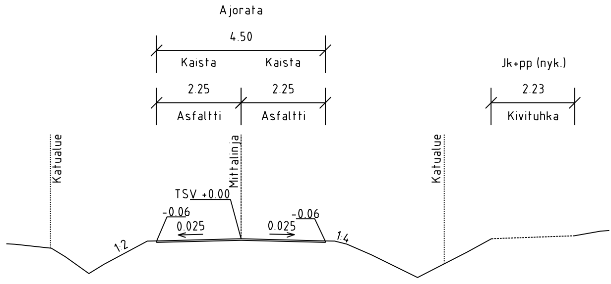
TYYPPIPOIKKILEIKKAUS G-G 1:100
