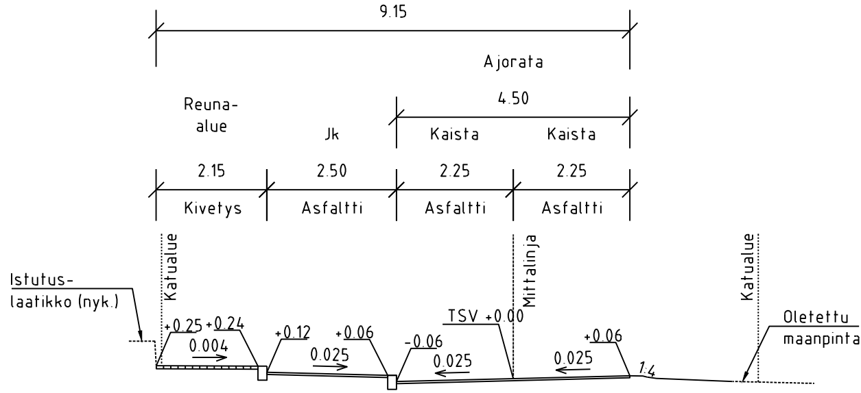
TYYPPIPOIKKILEIKKAUS D-D 1:100
