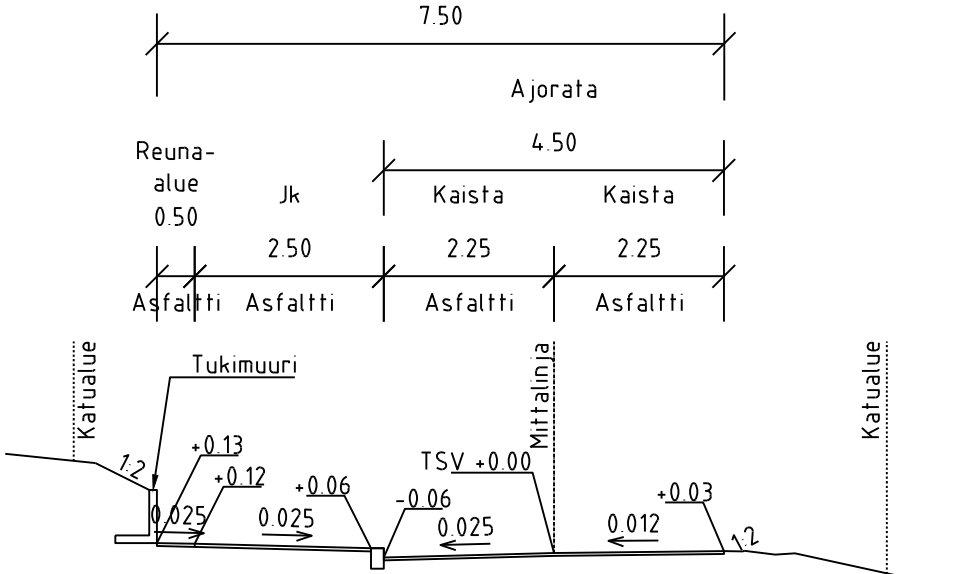
TYYPPIPOIKKILEIKKAUS E-E 1:100
