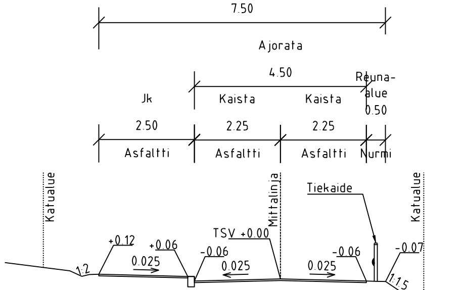
TYYPPIPOIKKILEIKKAUS F-F 1:100
