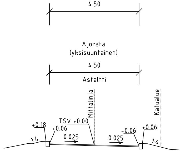
TYYPPIPOIKKILEIKKAUS A-A 1:100
