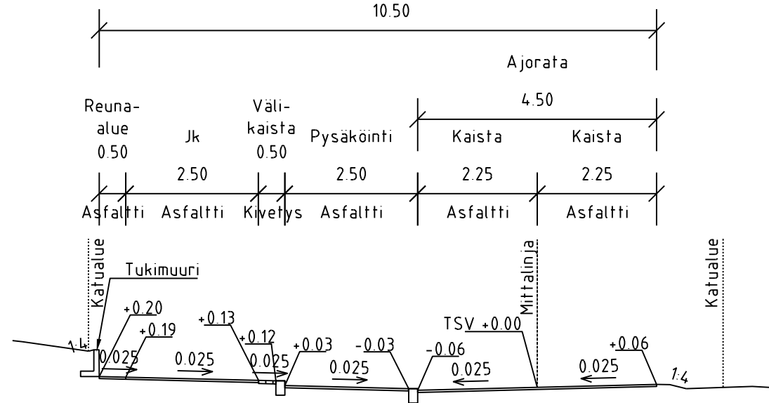
TYYPPIPOIKKILEIKKAUS C-C 1:100
