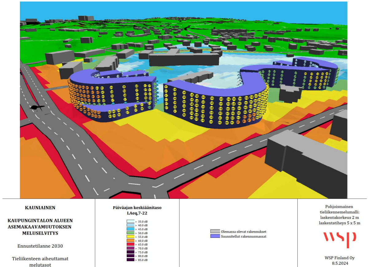
Kuva 7. Ote Kauniaisten kaupungintalon alueen meluselvityksestä (WSP Finland Oy, 2024).
