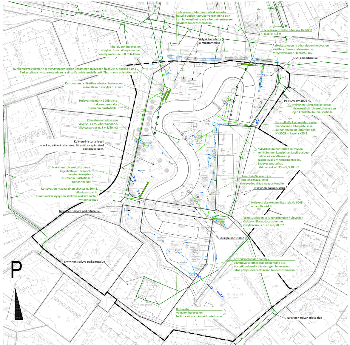
Kuva 15. Ote hulevesiselvityksestä (Sweco Finland Oy, 2024).
