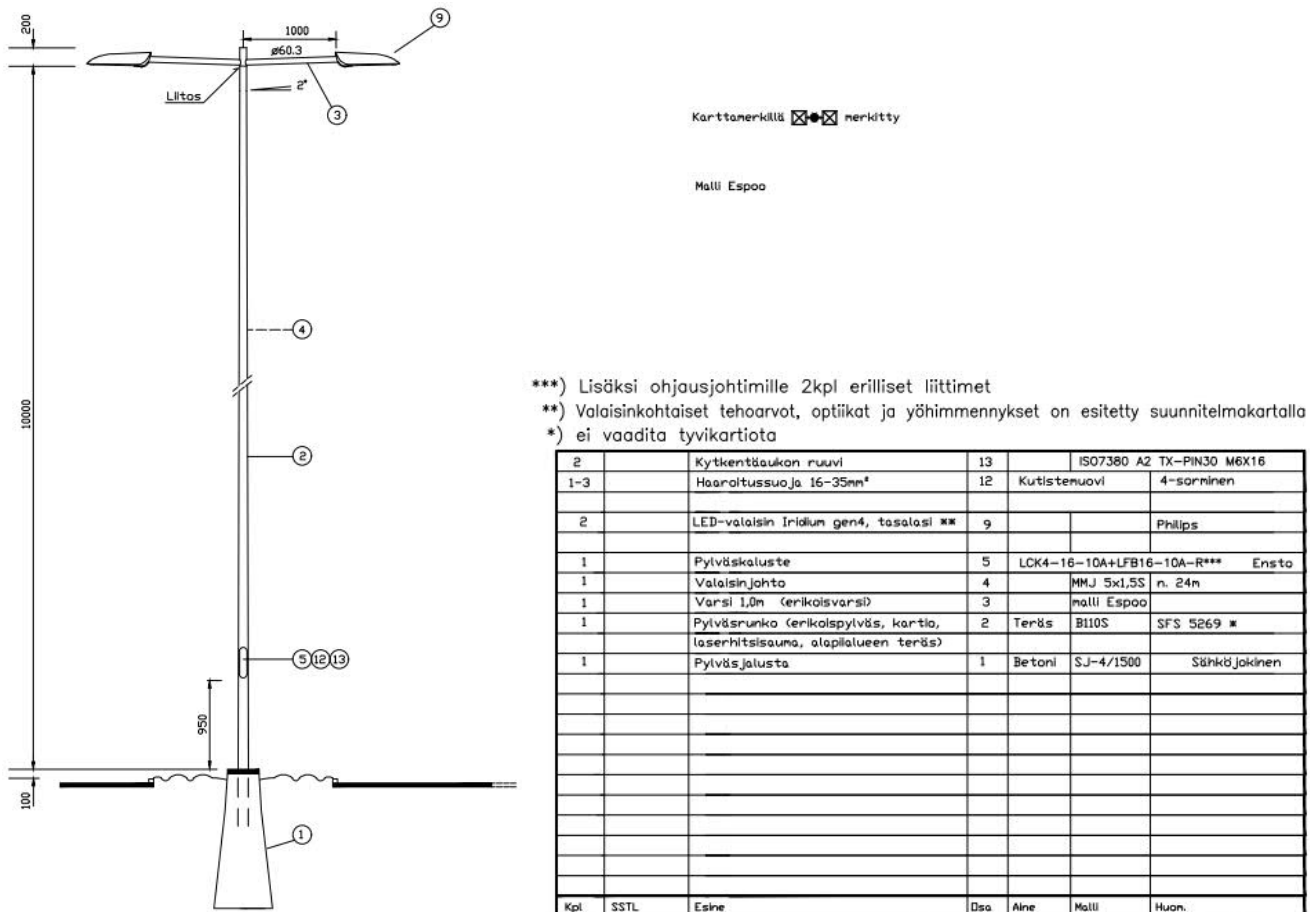
Kuva 6. Esimerkki liitepiirustuksesta. Pylvästyyppe malli Espoo, 10 m, kaksivartinen.
