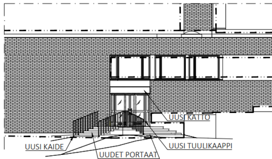
ETELÄPUOLEN TUULIKAAPIN SIVUKUVA
