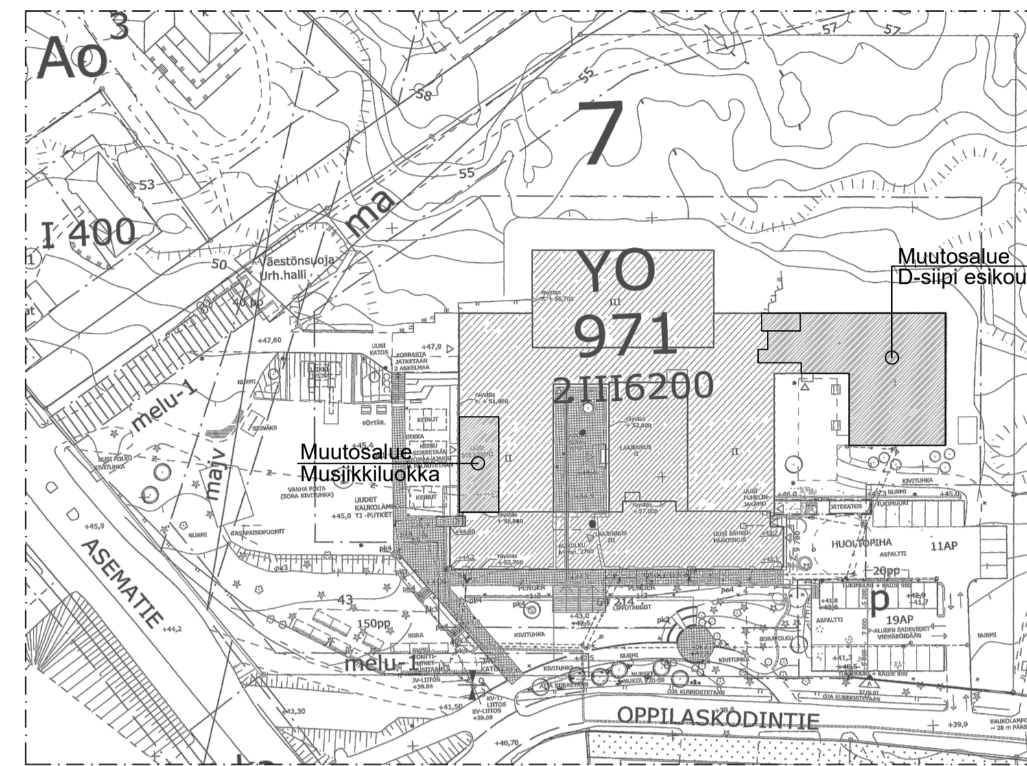
Situatiopiirros 1:1000
